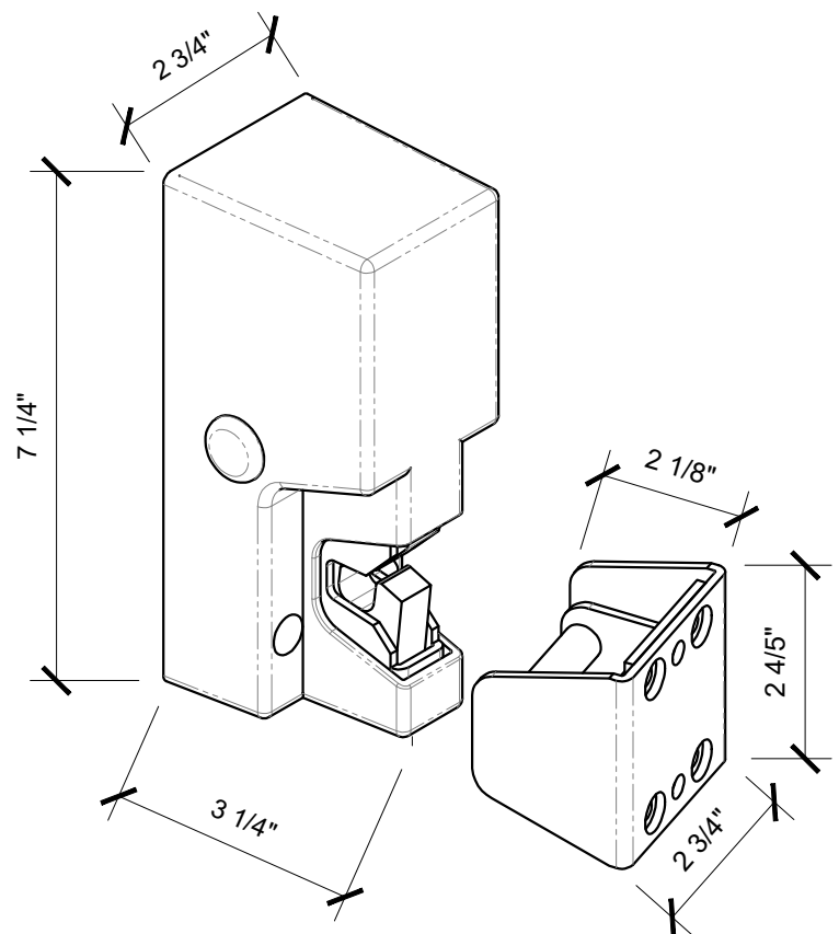
2 LATCH DETAIL C601 SCALE: NTS
